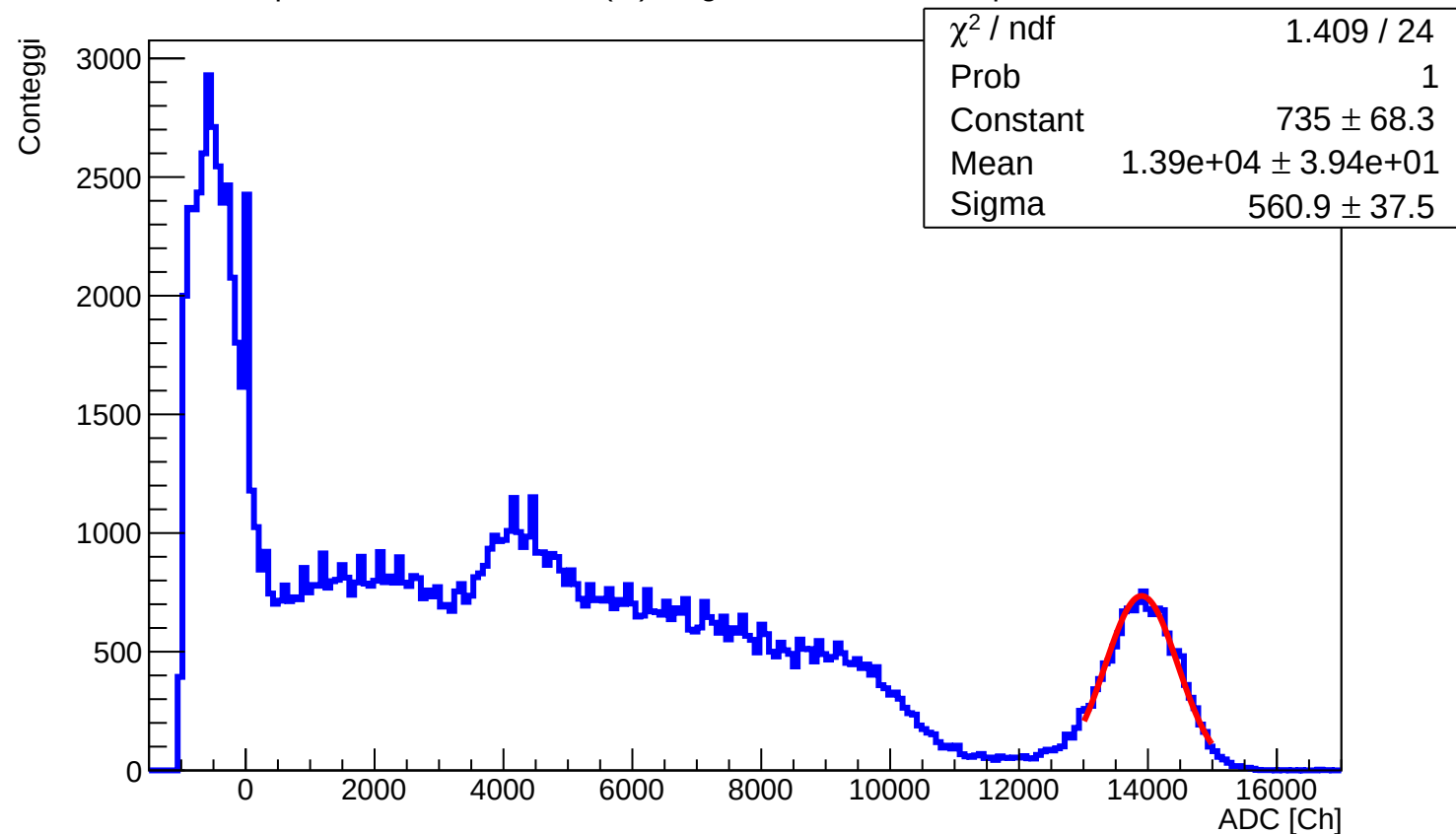
Spettro del ^{137}\text{Cs} con CsI(Tl), soglia a 50 mV e fit sul picco fotoelettrico
